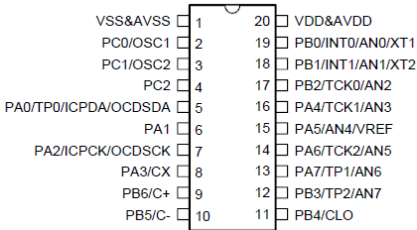
图 2-3 SOP20/SSOP20 引脚排列图
