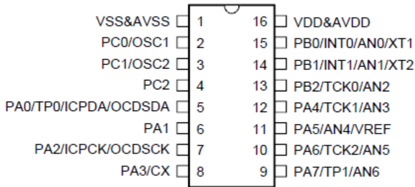
图 2-2 NSOP16 引脚排列图
