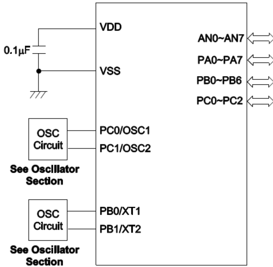
图 8-1 应用电路
