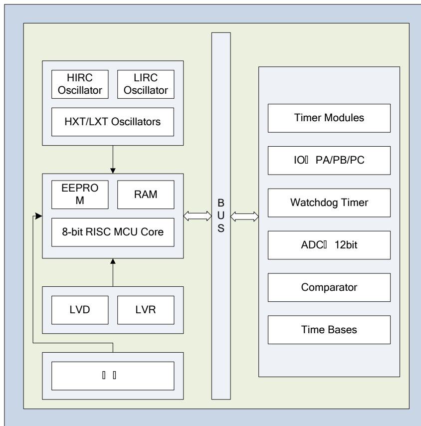
图 2-1 功能框图
